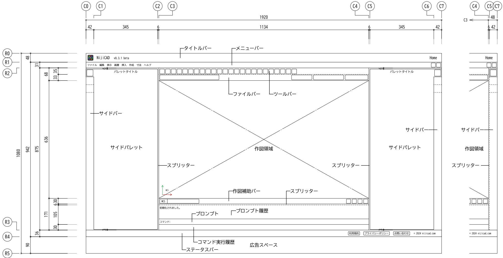
全体姿図 S=1/10 (サイドパレット初期状態)
